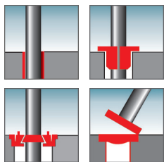
Mögliche Bodenhalterungen
